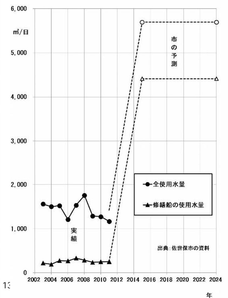
図7(2) SSKの使用水量の実績と市予測
