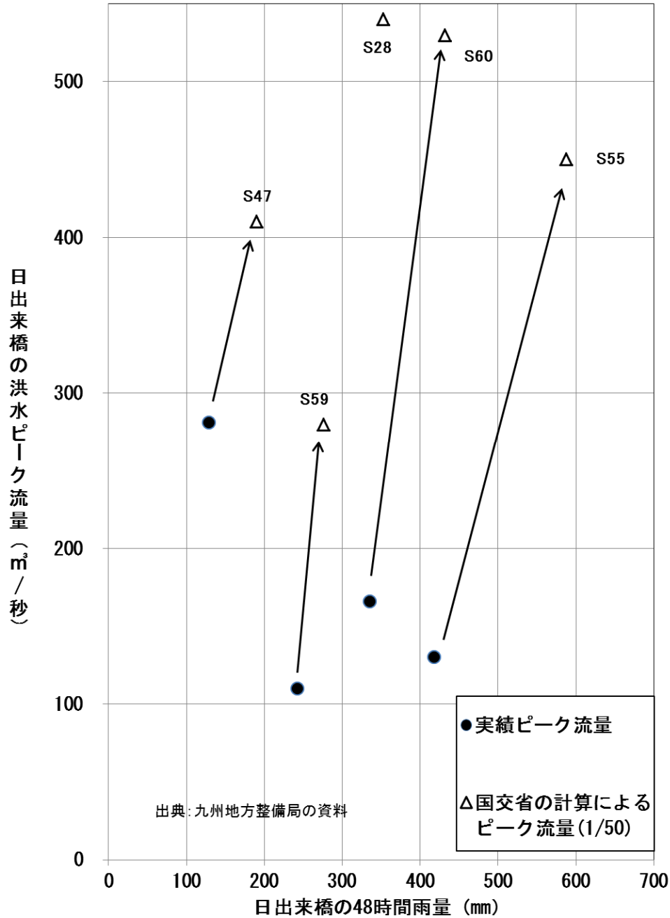
図1 城原川の雨量と洪水ピーク流量の関係 (1)
