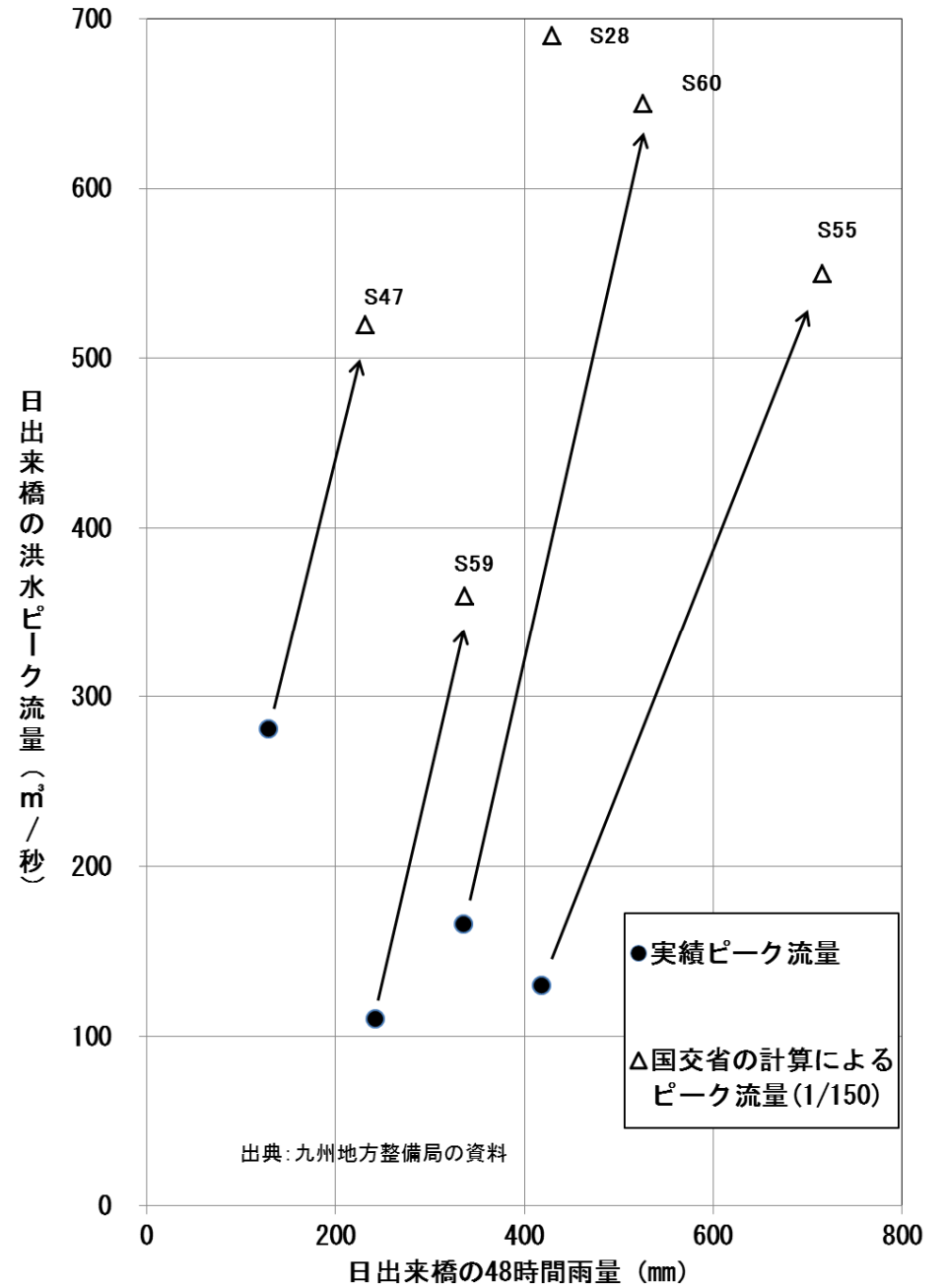
図2 城原川の雨量と洪水ピーク流量の関係 (2)
