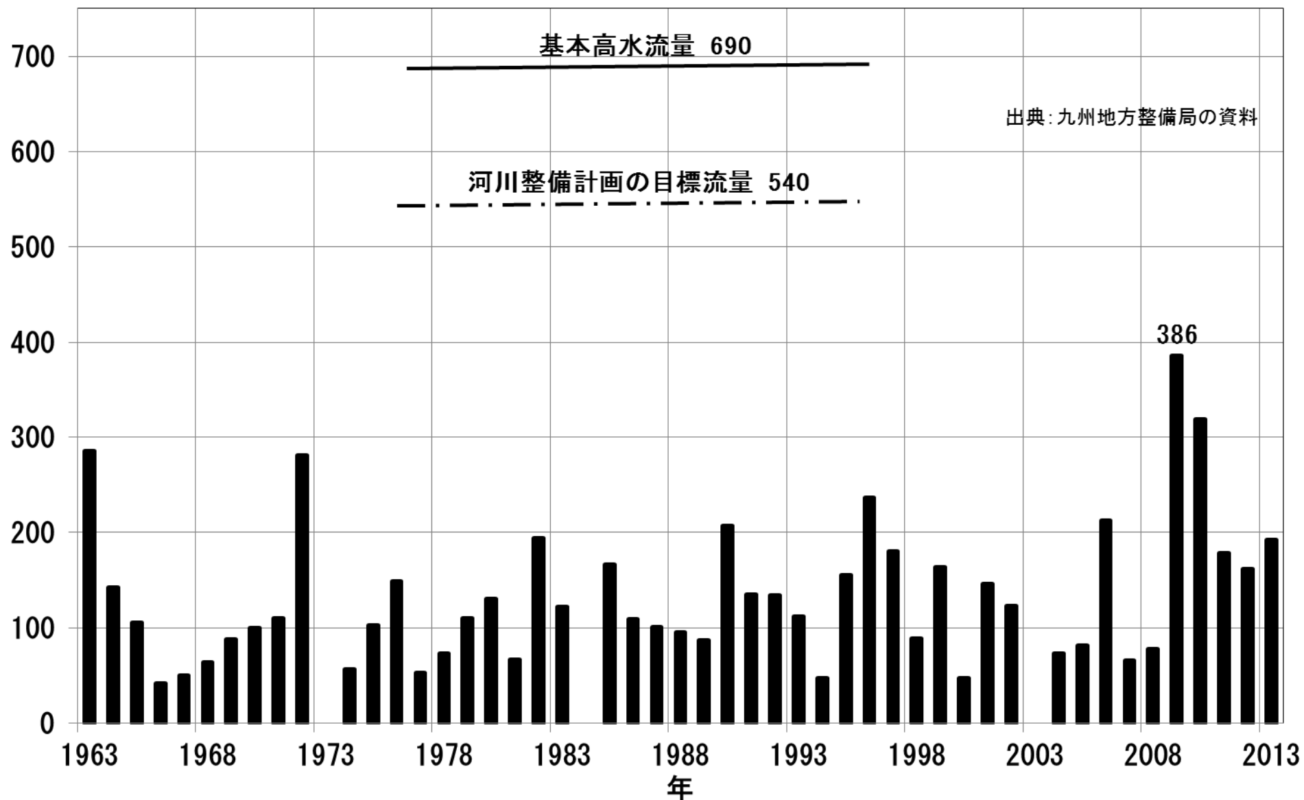
図3 城原川・日出来橋の年最大観測流量の推移
