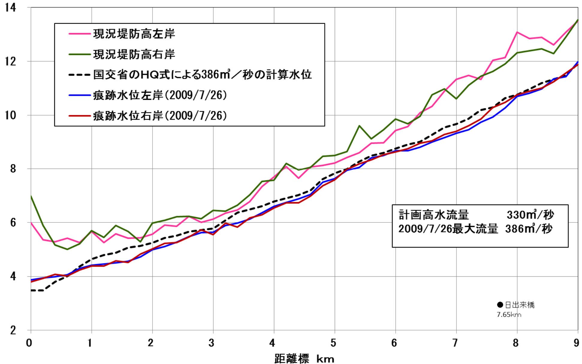
図4 城原川の国交省計算水位と洪水痕跡水位
