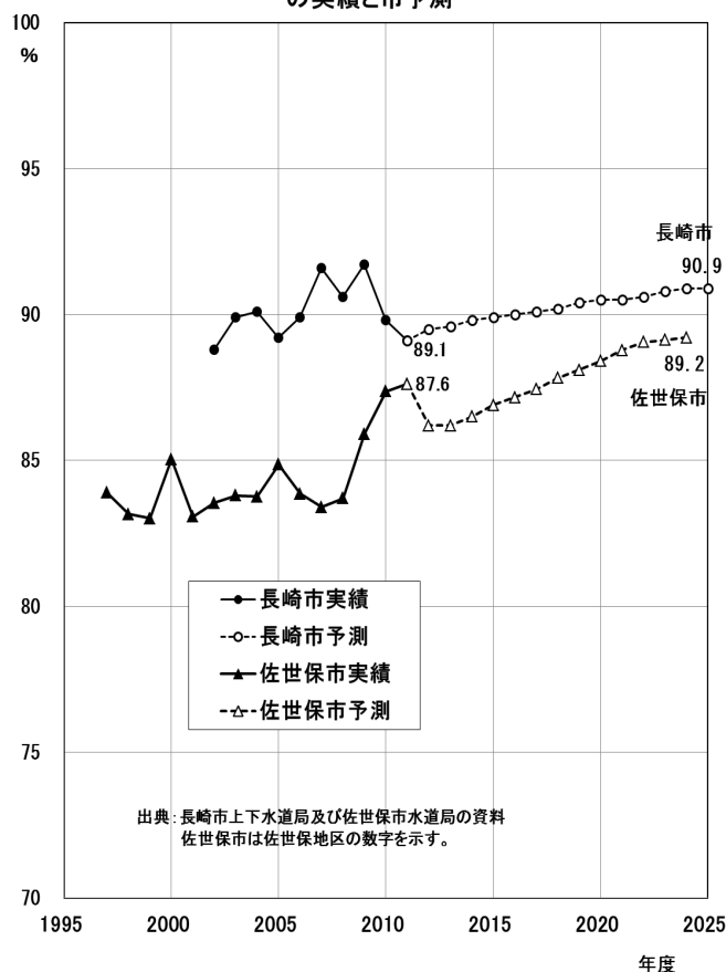
図7 長崎市及び佐世保市水道の有収率の実績と市予測
