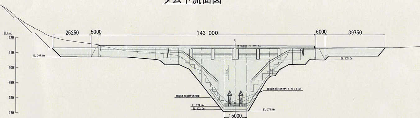
ダム下流面図
