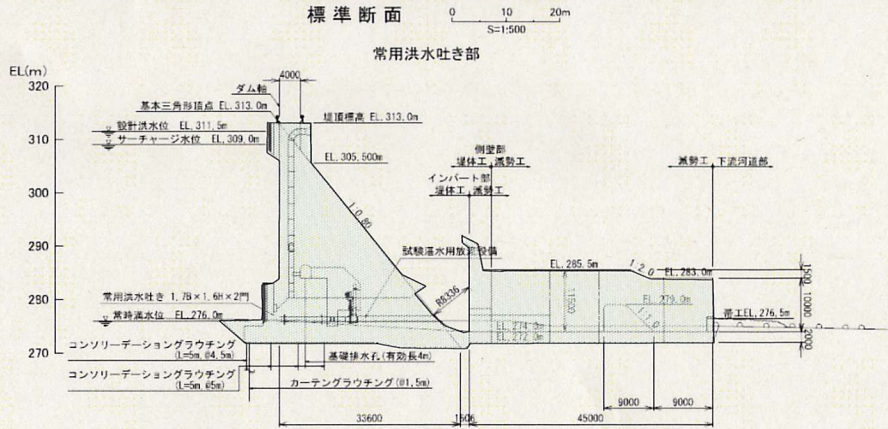
越流部標準断面図
