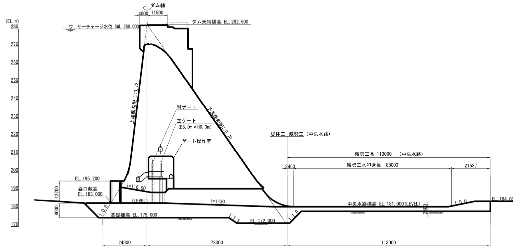
常用洪水吐き
