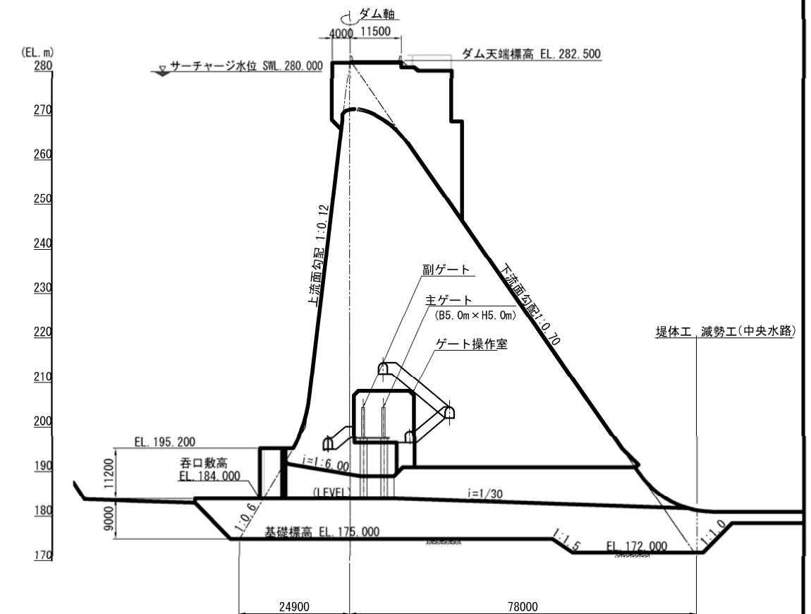
河床部放流設備（右岸）
