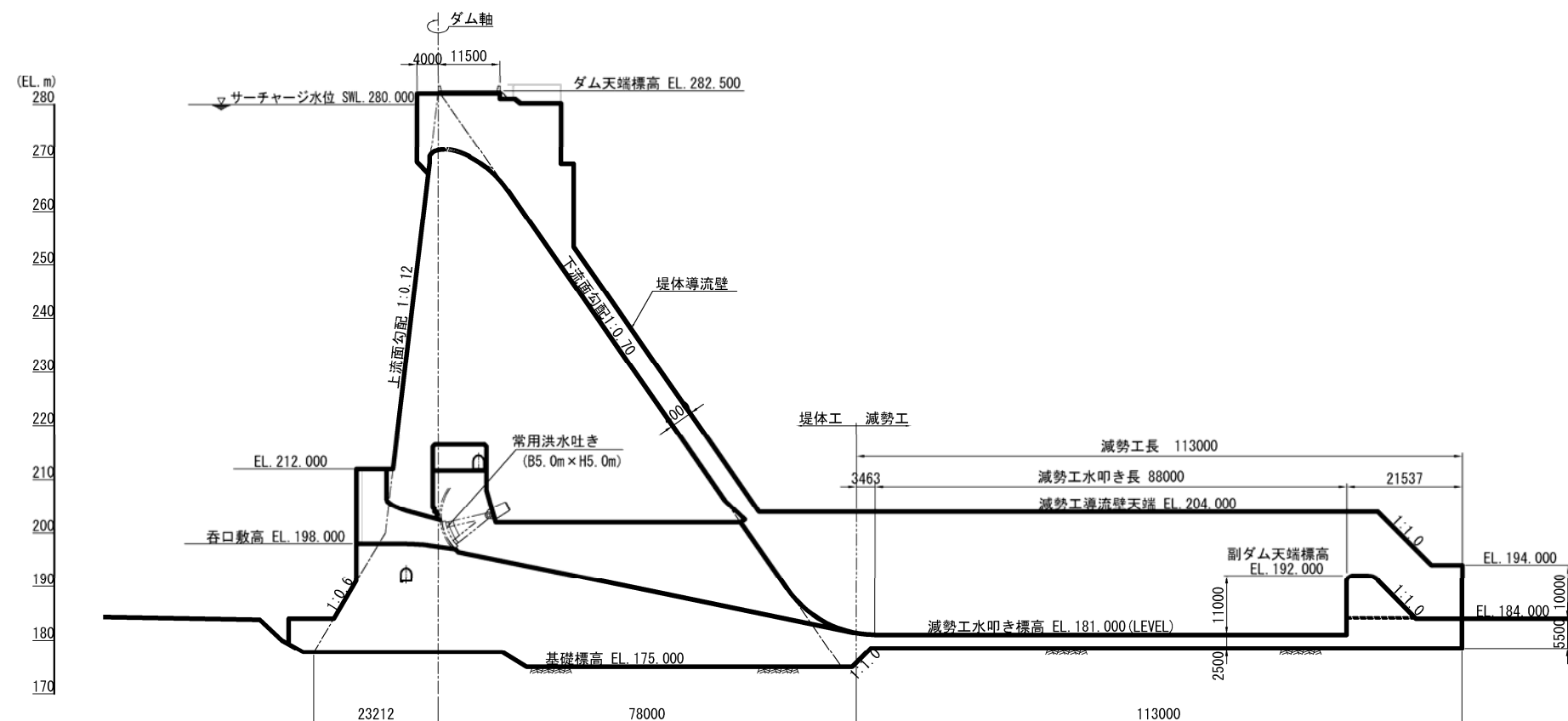
常用洪水吐き
