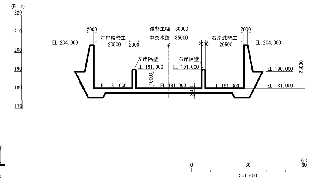
減勢工標準断面図
